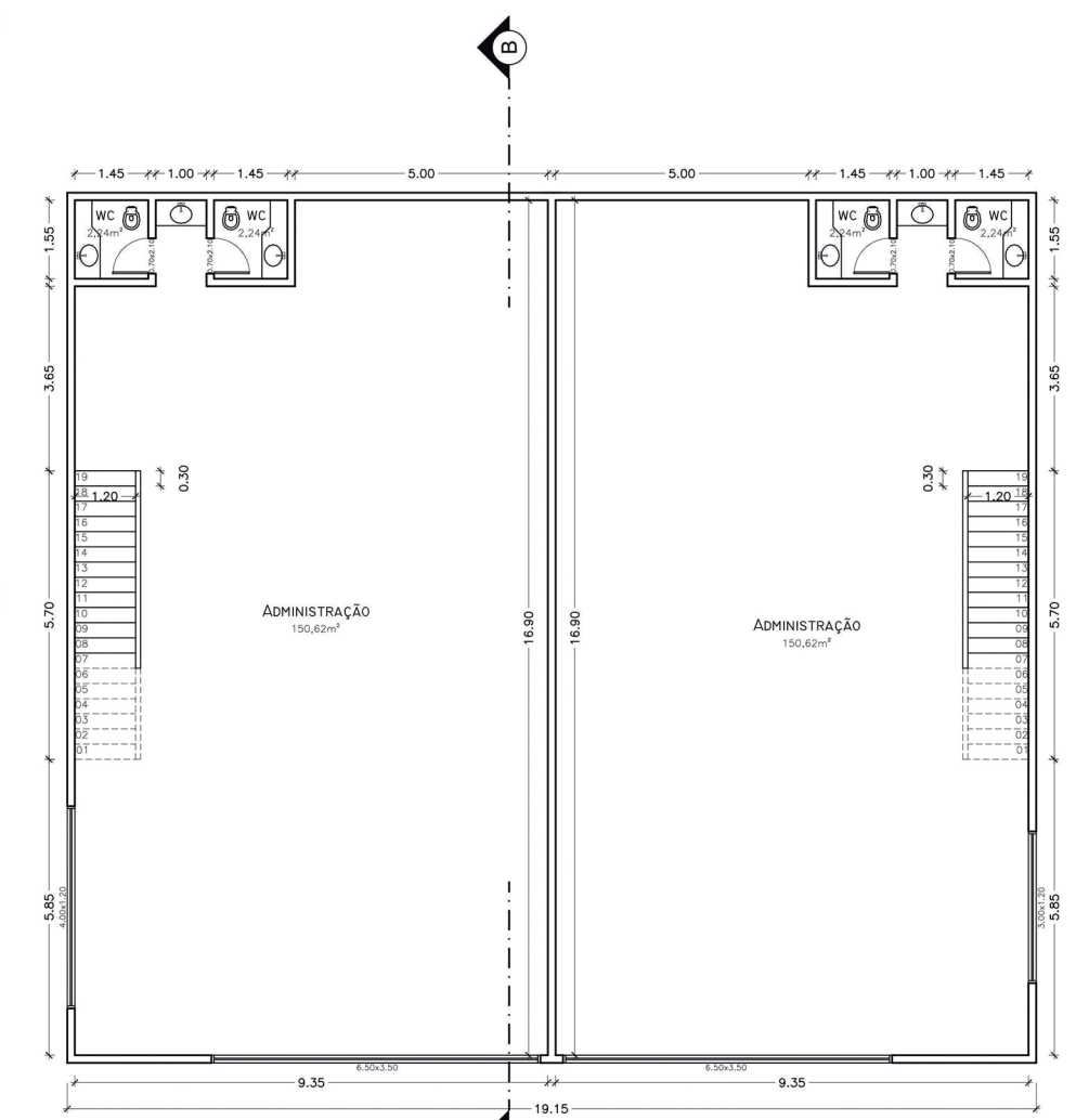
PLANTA BAIXA SEGUNDO PAVTO. 1:100
